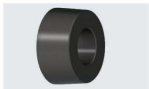
Zentrierhülse für BMW-Sonderfahrzeuge Mittenloch Ø 80–83,7/81,5 mm Bestellnummer: 1 692 502 037
