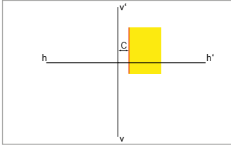
Matrix-Scheinwerfer rechts
