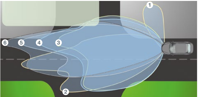
Beleuchtungssituationen mit moderner Lichttechnik: ① Abbiegelicht ④ Stadtmodus ② Dynamisches Kurvenlicht ⑤ Überlandmodus ③ Schlechtwettermodus ⑥ Autobahnmodus
