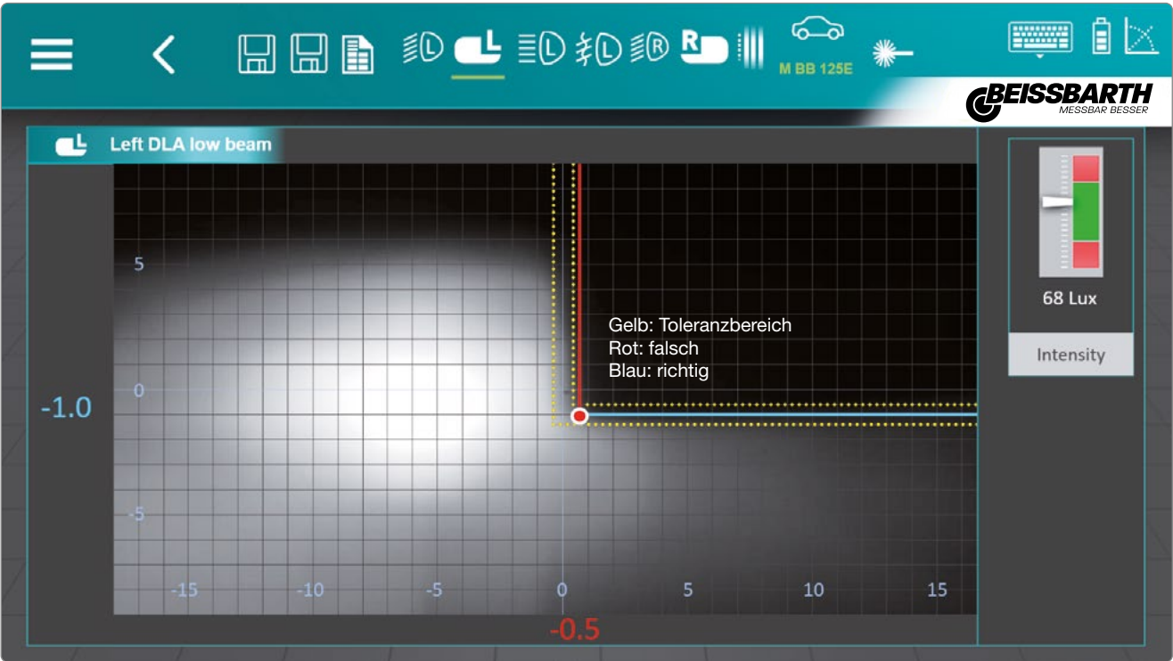
Einstellung eines Scheinwerfers mit Fernlichtassistent DLA (Testbildansteuerung über die Steuergeräte-Diagnose am Fahrzeug*)
